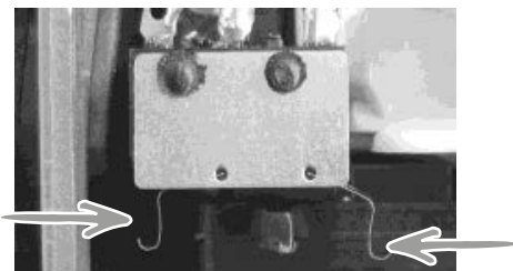
Comutator de protecție al diafragmei neactivat. (Mod de operare normal.)
