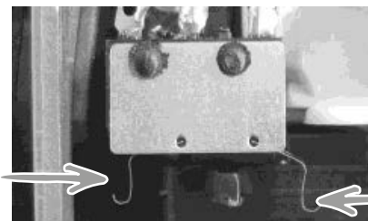
Diafragma de proteção interruptor não ativado. (Modo de funcionamento normal)
