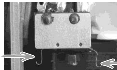
Diafragmabeschermings -schakelaar niet geactiveerd. (Normale gebruiksmodus.)
